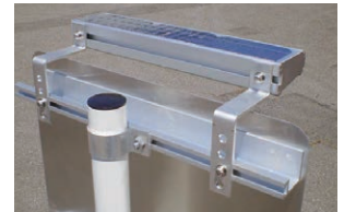
標識用取付金具
